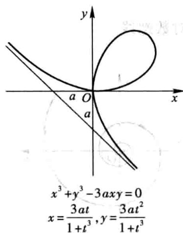
(6) 笛卡儿叶形线
