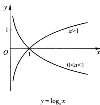
对数函数
