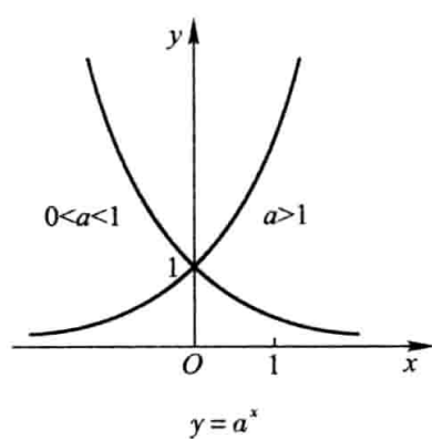
指数函数
