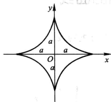
(7) 星形线(内摆线的一种)
