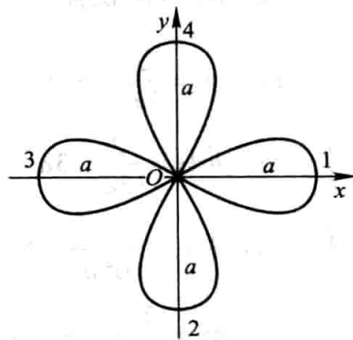
(18) 四叶玫瑰线
