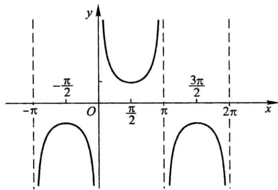
y = \csc x
