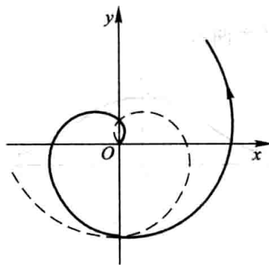
(10) 阿基米德螺线
