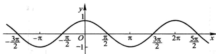
y = \cos x
