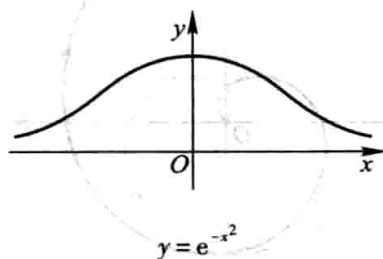
(3) 概率曲线
