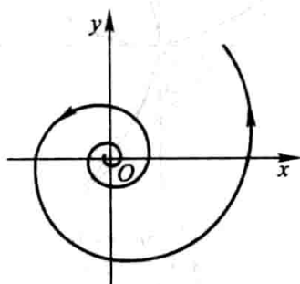
(11) 对数螺线
