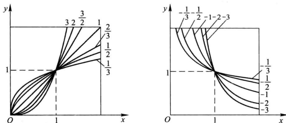
幂函数
