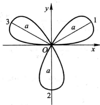
(16) 三叶玫瑰线
