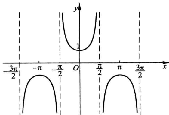
y = \sec x
